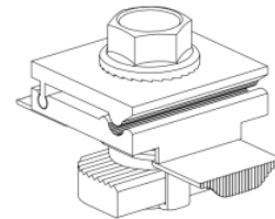
12 Ground lug 1 | 3010407
